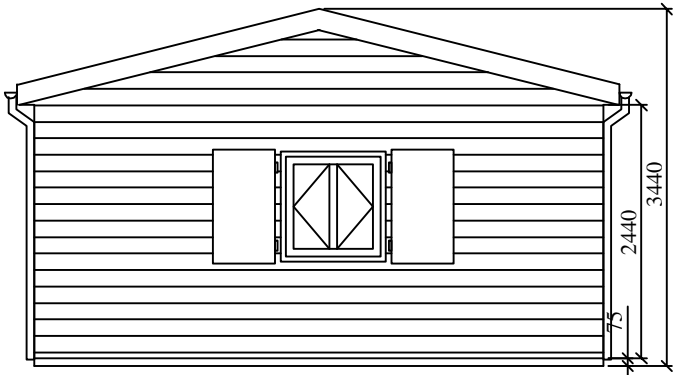
END ELEVATION
