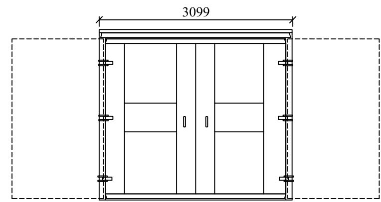
END ELEVATION
