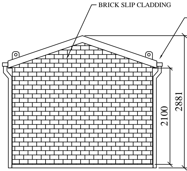
END ELEVATION
