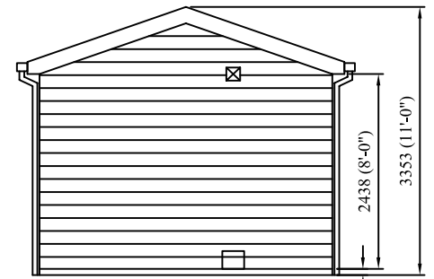
END ELEVATION
