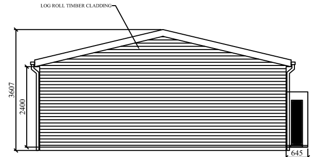
SSE ELEVATION
